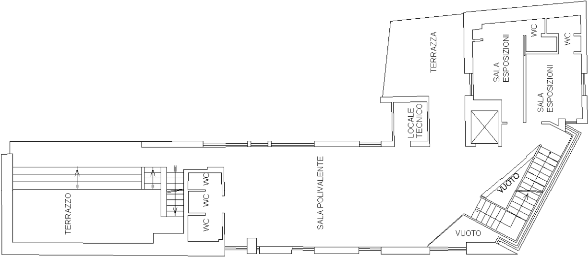
PIANO PRIMO H=2.80
